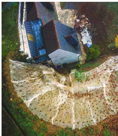
LITE-NET als Anwachshilfe (Aufnahme von oben)
